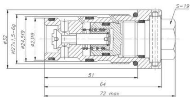
Рисунок 1 Гидрозамок ввертный ГЗВ.00.000
