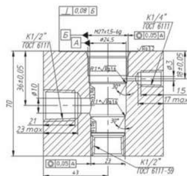
Рисунок 2 Присоединительные размеры монтажного отверстия
